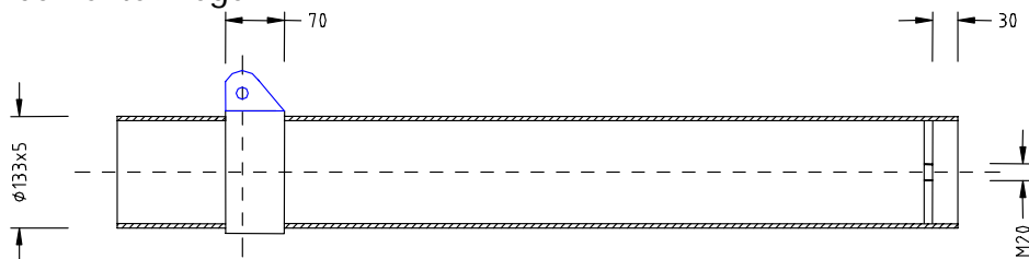
Mastfuß
